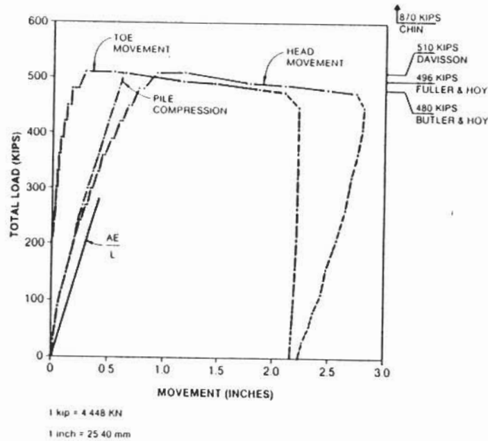
FIG. 7. Pile A-4
