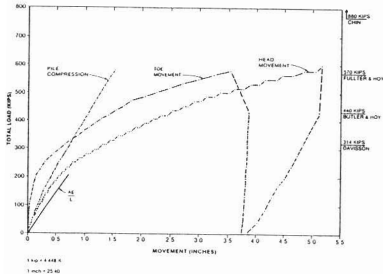
FIG. 8. Pile B-2
